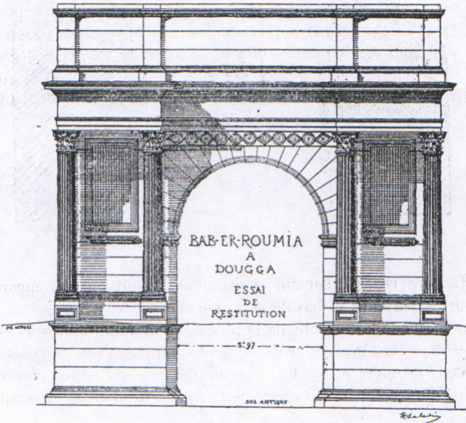
— Élévation restituée de Bab-er-Roumia.
